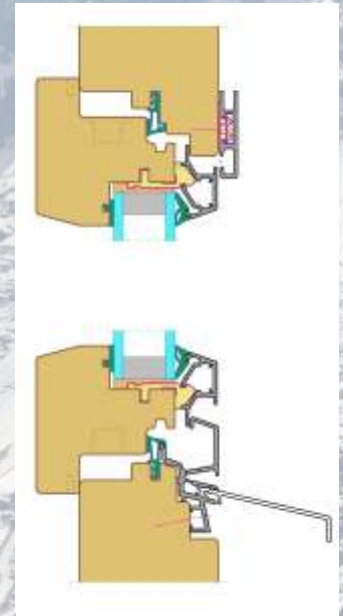
Holz/Metall-Fenster Sirius L
